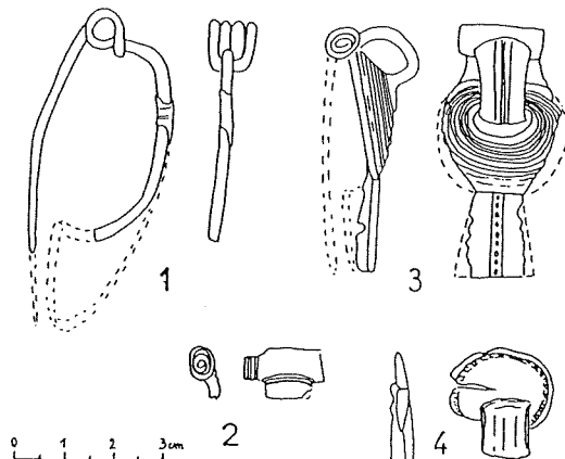
FIG. 7. ... fibules
